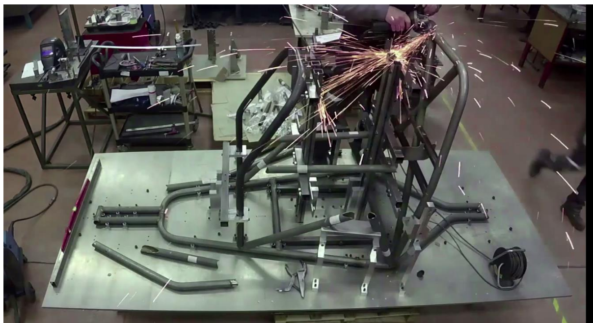
Soudure d'un châssis XC Cross Car
