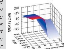
Graphique caractérisant un pneu (adhérence disponible) Graph showing available traction of tyre
