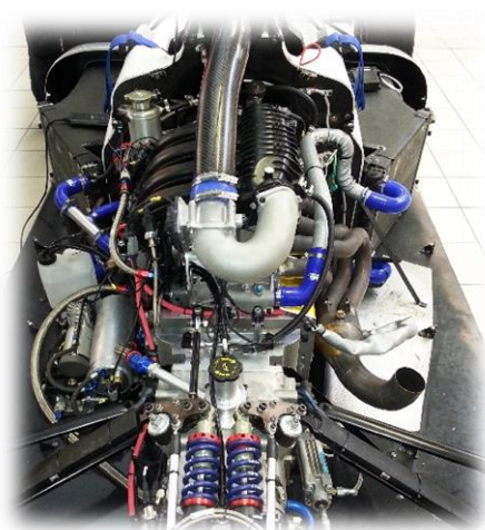
Vue de dessus du moteur Renault F4.
