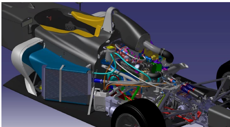
Implantation du moteur Renault 1.3T dans la F4
